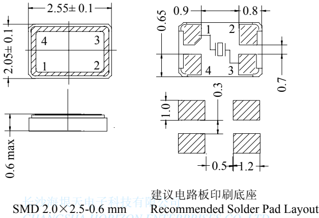
外形尺寸(单位:毫米) Figure and Dimensions(Unit: mm)
