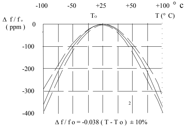
长沙海根天电子科技有限公司 频率温度曲线图 Frequency Temperature Curve CHANGSHA HORIZON ENTERPRISES CO.,LTD.
